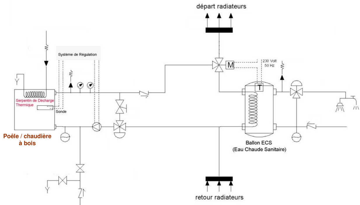
Schéma de principe d'une installation type
